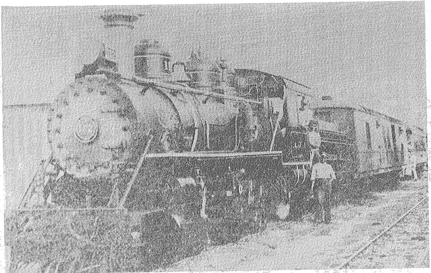
La máquina Núm. 112 del Tren de Pasajeros desde Ponce, Santa Isabel, Salinas hasta Guáyama. Las máquinas de pasajeros y las de carga (Aguirre) son casi iguales excepto la diferencia en las ruedas. Las de carga (Aguirre) son pequeñas, lentas pero muy poderosas. Las de pasajeros son ruedas enormes, altas, para mucha velocidad. Note la enormidad de esta máquina por las ruedas altas; está tirando de vagones de pasajeros; de 3ra. clase con asientos de madera, de 2da. clase con asientos de pajilla y la 1ra. clase los llamaban Pulman con asientos de cuero y otras comodidades.
